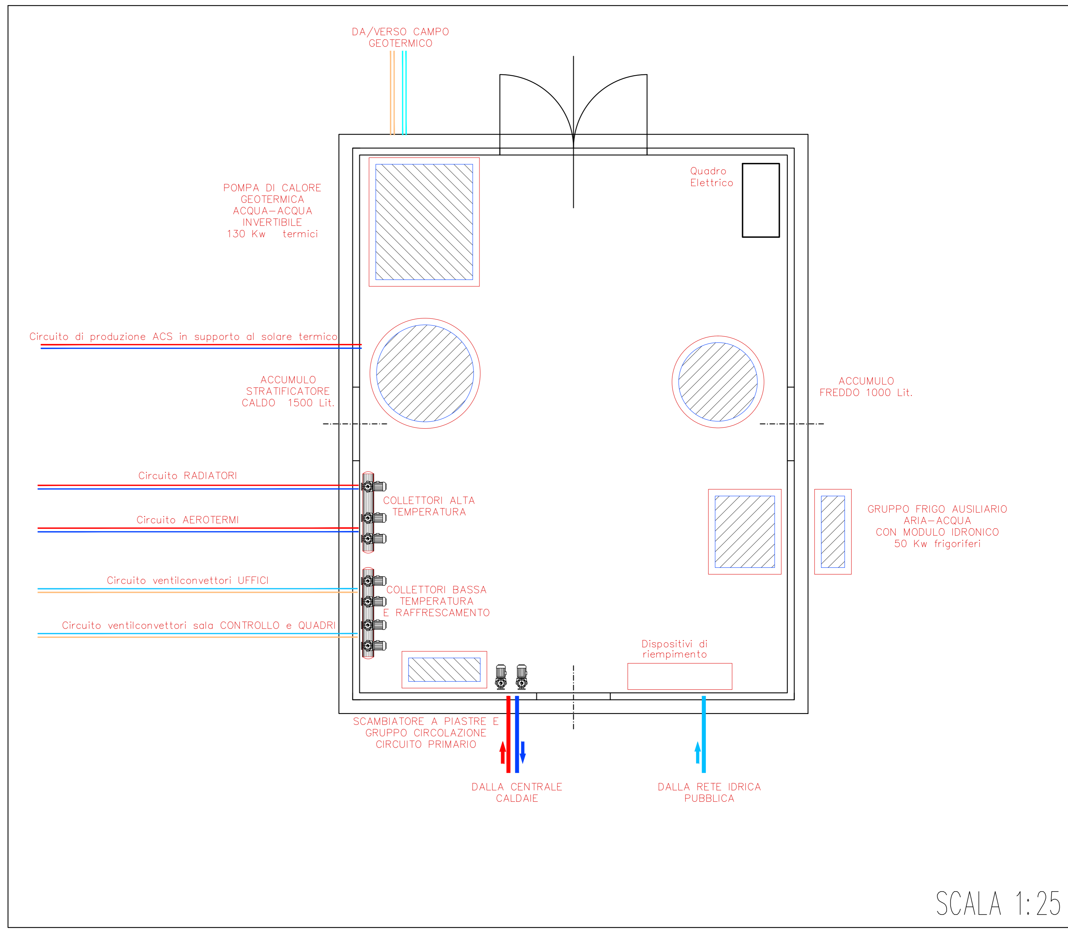
LOCALE SOTTOSTAZIONE HVAC Vista in Pianta
